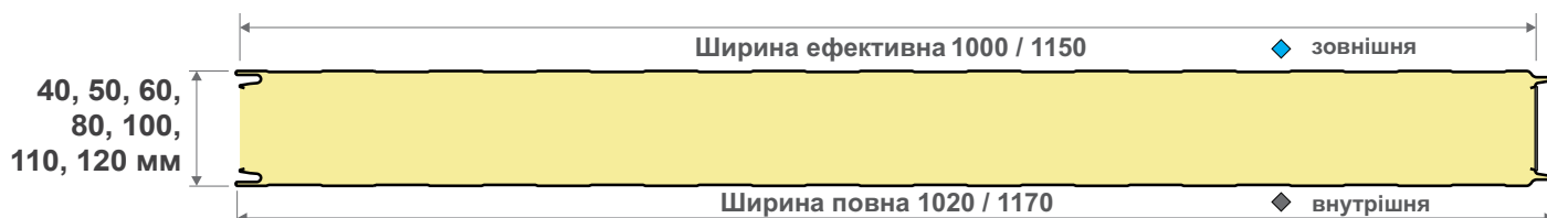
Поперечний переріз
